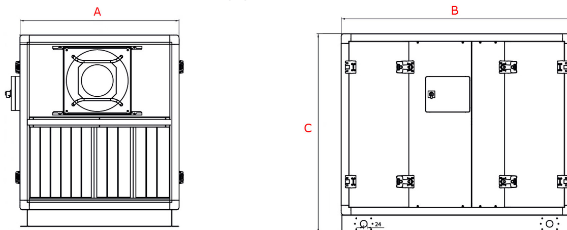
GLOBAL PX (FW)
